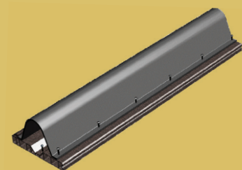
POLY PILLOW EN BASISPLAAT Aanbevolen bij al onze loopstelsystemen om de koe te helpen bij het positioneren en om de stal schoon en droog te houden.
